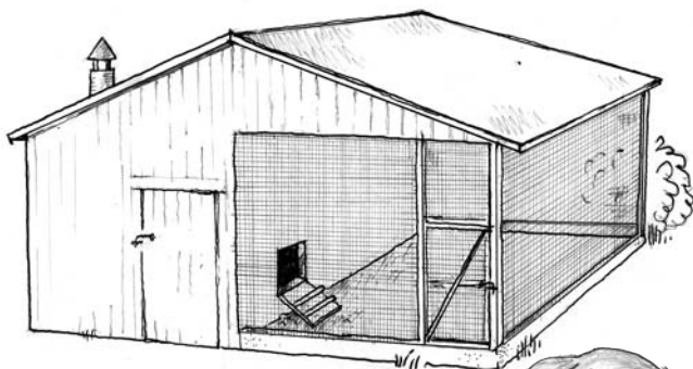
Figur 1. Exempel på uterum (veranda). Uterummet har tätt tak och väggar av sexkantnät med en maskstorlek på högst 19 mm. Nätet fästs vid en sockel som är nergrävd några dm i marken. Uterummet behöver inte vara inbyggt, som på bilden, utan kan likaväl vara en tillbyggnad.
