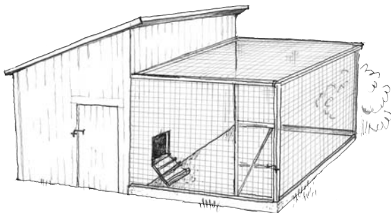
Figur 4. Inhägnaden har väggar av sexkantnät med en maskstorlek på högst 51 mm. Där så är praktiskt möjligt ska inhägnaden förses med ett nättak av nylonväv. Lösa nät av typen fruktnät ska helst inte användas.
